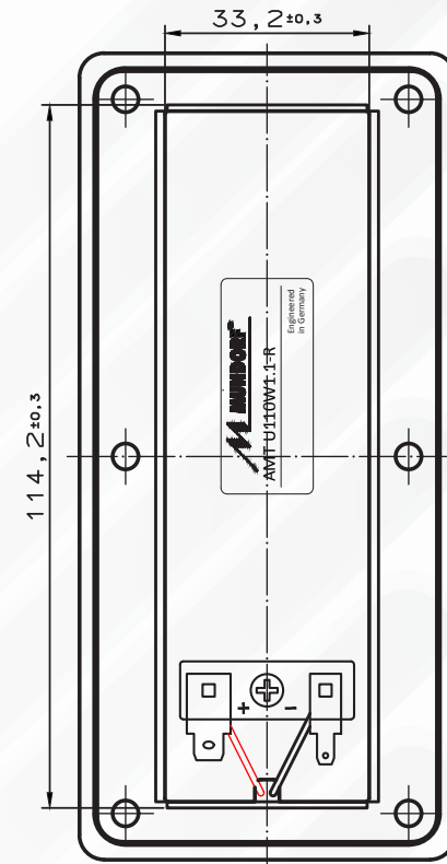
Ansicht Hinten
