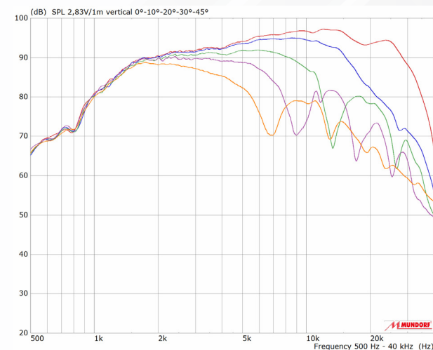
SPL Vertikal 0° - 10° - 20° - 30° - 45°
