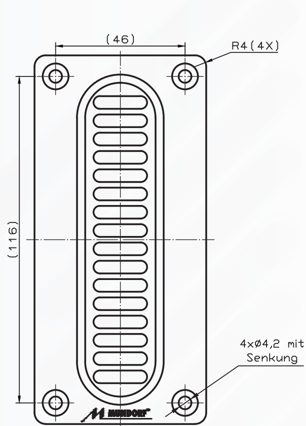
Ansicht Vorne
